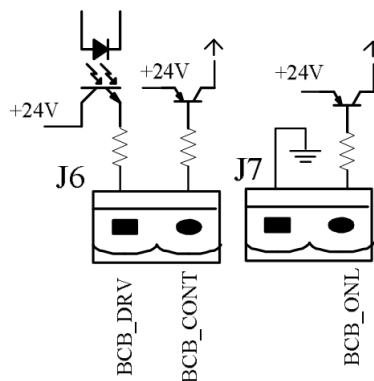
Рис. 1-16. Интерфейс ВСВ
