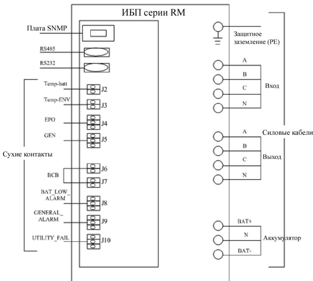
Рис. 1-21. Схема установки
